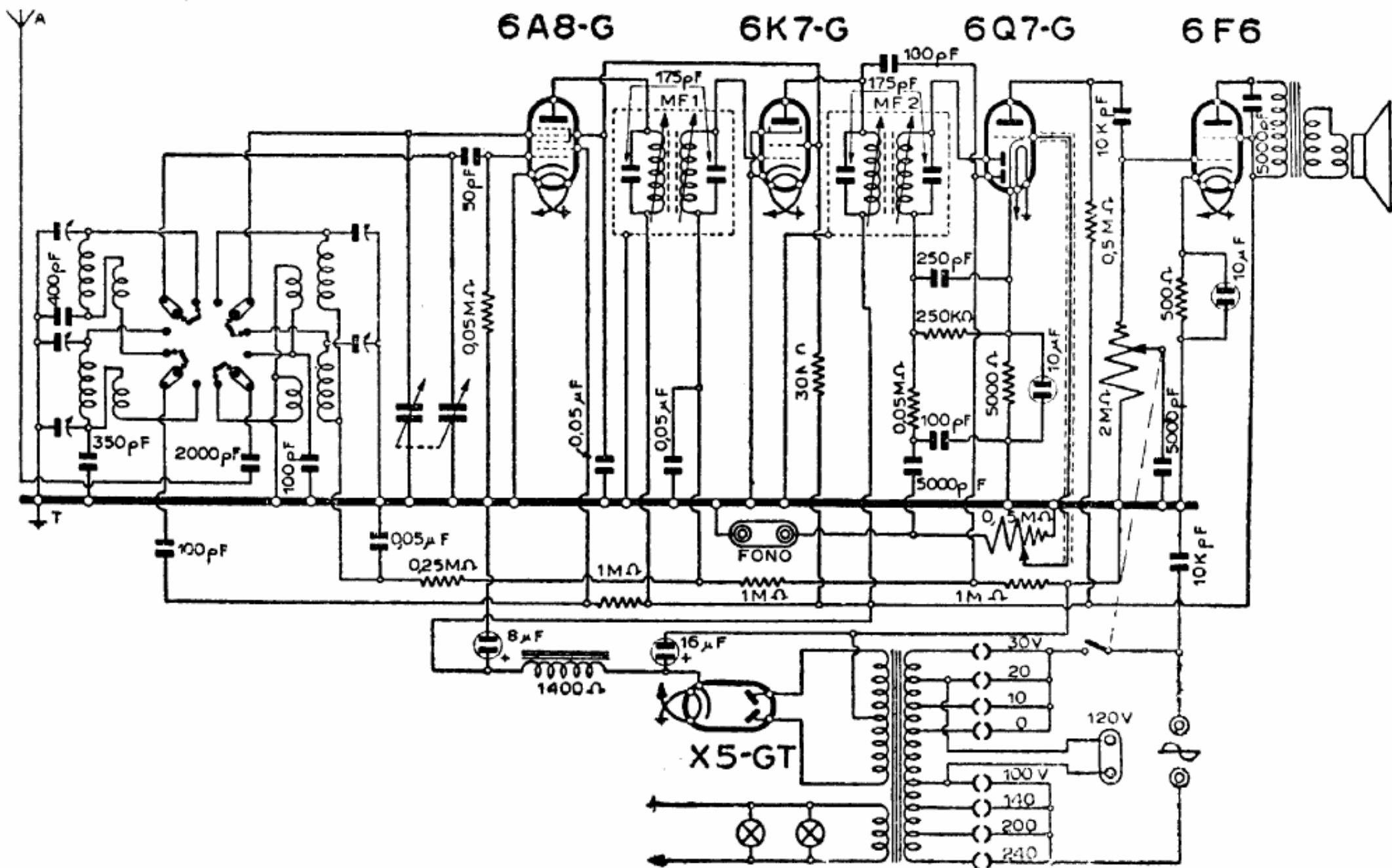
Lo schema elettrico dei modd. «504» • «509» Siare (telai 2522 - 2524).
